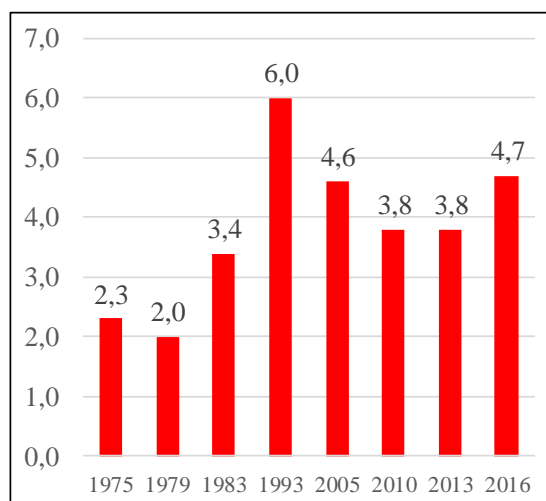
Figur 4: Ledighetstopper
